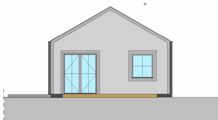
ELEWACJA WSCHODNIA
