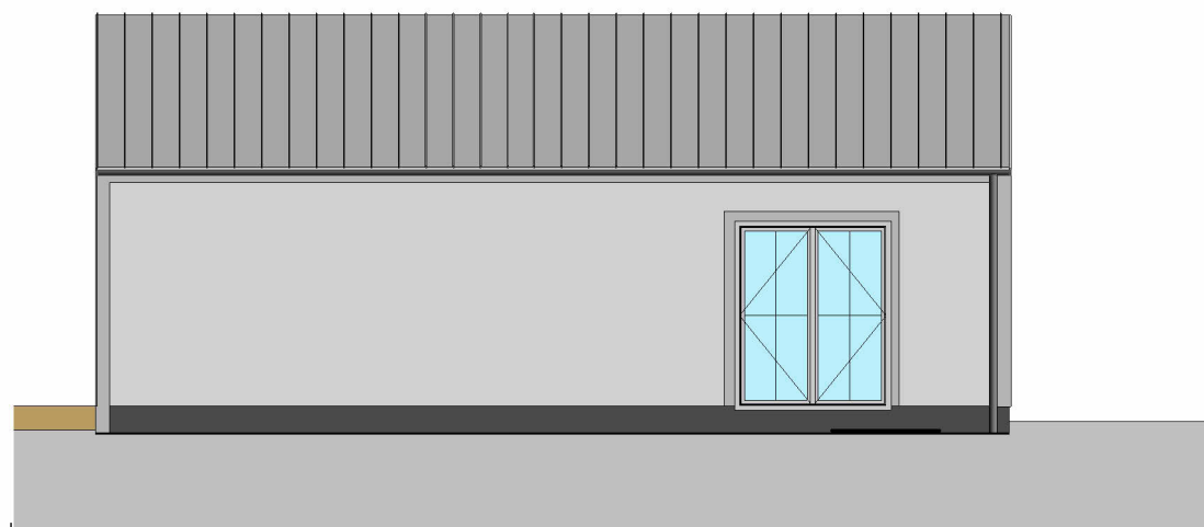
ELEWACJA PÓŁNOCNA
