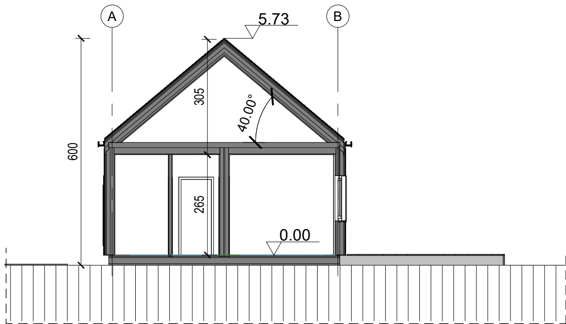
PRZEKRÓJ A-A
